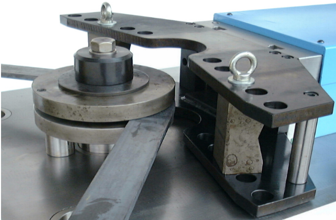
Prípravok na ohýbanie plochej ocele do max. bending on edge up to 60 x 15 mm
