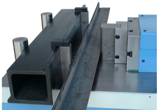
Vyrovňavací prípravok nosičov do výšky straightening of H-beam , T-profile and other profiles up to 250 mm
